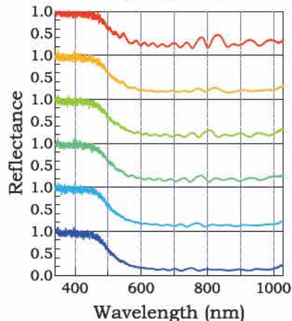
図2 内部構造の異なるポーラスアルミナ箔からの可視光反射率スペクトル。
