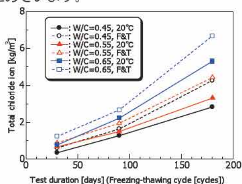
凍結融解作用を受けるコンクリートの塩化物イオン浸透性
