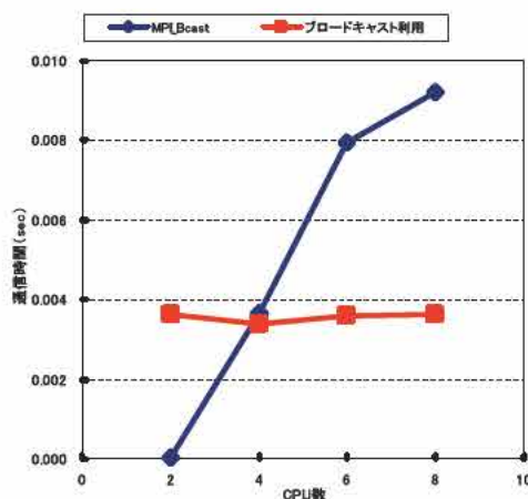
図 2. MPI 集団通信の性能改善結果
