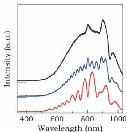
図1 アルミホイル(一番上)と内部構造の異なるポーラスアルミナ箔(下の二つ)からの可視光反射スペクトル。
