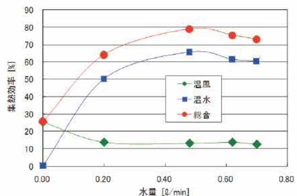
図 集熱効率の変化（屋外実験・風量 0.4 [m/min] 一定）
