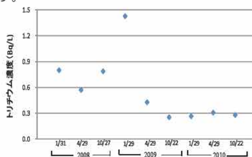
図1 尾駸沼で採取した水試料のトリチウム濃度
