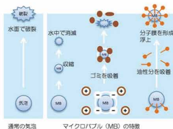
マイクロバブルの消失過程
